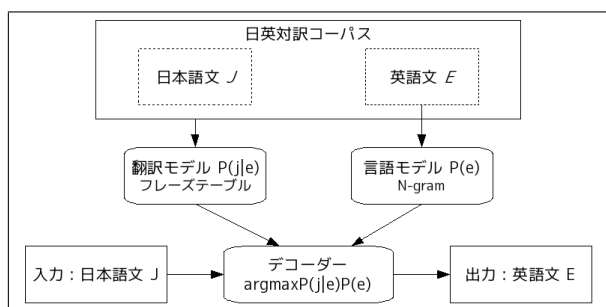
図 1 日英統計翻訳の枠組
