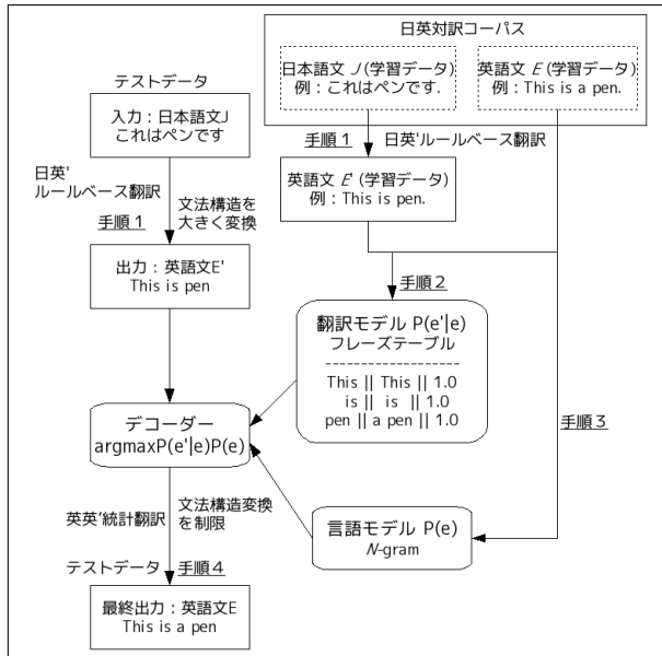
図2 提案手法の枠組
